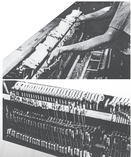
วิธีการยก Spinet Action ออกจากตัวถังเปียโนต้องใช้เชือกหรือลวดมัด Butt wire ไว้ก่อนเป็นการป้องกันการเสียหายของ Butt
